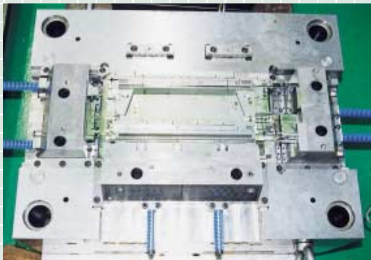
OA関連ホットランナーハイサイクル金型
